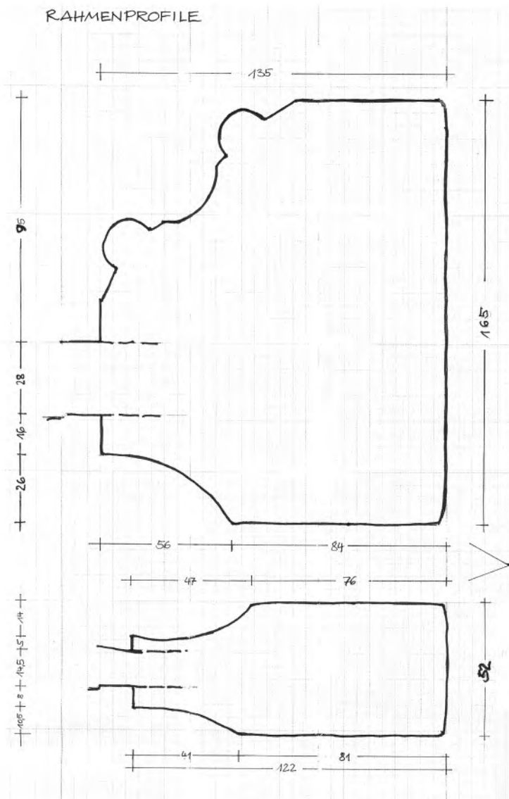
Abb. 37 Rahmenprofile (Zeichnung B. Hartwieg)
