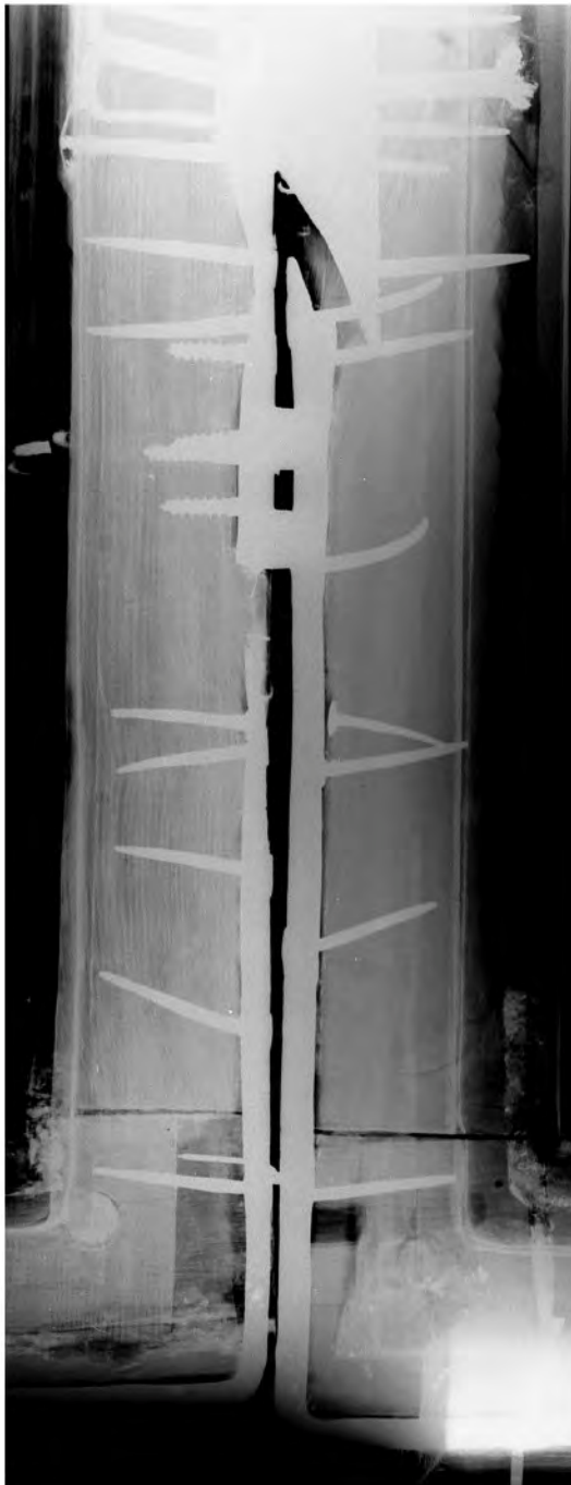
Abb. 41 a,b: Eckverbindungen Mitteltafel und Innenflügel, Röntgenfotos
