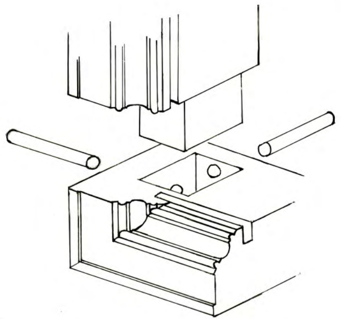
Abb. 40: Schemazeichnung: Eckverbindung Mitteltafel
